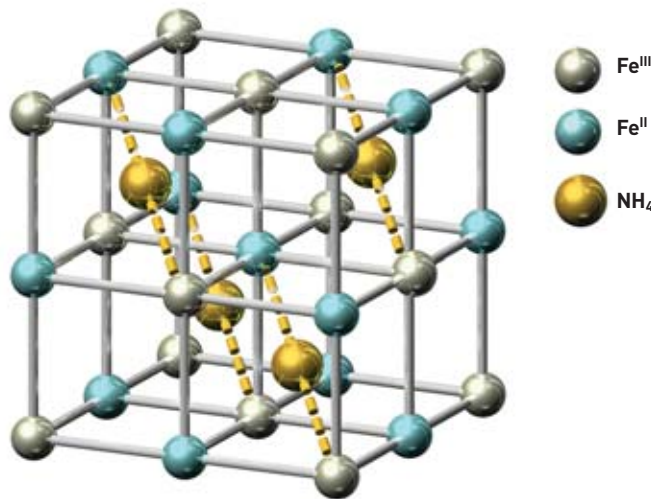
Figure 1. Ferrocyanure (II) d'ammonium ferrique (III) [\text{NH}_4]_2 \text{Fe}^{3+} \text{Fe}^{2+} (\text{CN})_6] ou AFCF, commercialisé sous le nom de "sel de Giese". Ce dérivé du bleu de Prusse permet de réduire fortement la contamination en césium de la viande et du lait, l'ion \text{Cs}^+ prenant la place du \text{NH}_4^+ .
