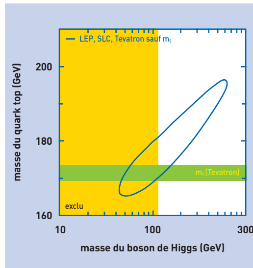
Figure 5. Comparaison des mesures expérimentales et des prédictions théoriques qui sont fonction des masses du boson de Higgs ( M_H ) et du quark top ( M_{top} ). Dans le plan (M_H, M_{top}) , le contour issu des mesures de précision (hors mesure directe de M_{top} ) et tenant compte des incertitudes expérimentales (ellipse) est comparé à la mesure directe de M_{top} (bande horizontale). Les deux régions se recouvrent pour des valeurs de M_H entre 50 et 200 GeV environ. La bande verticale est la région exclue par les recherches directes du boson de Higgs.
