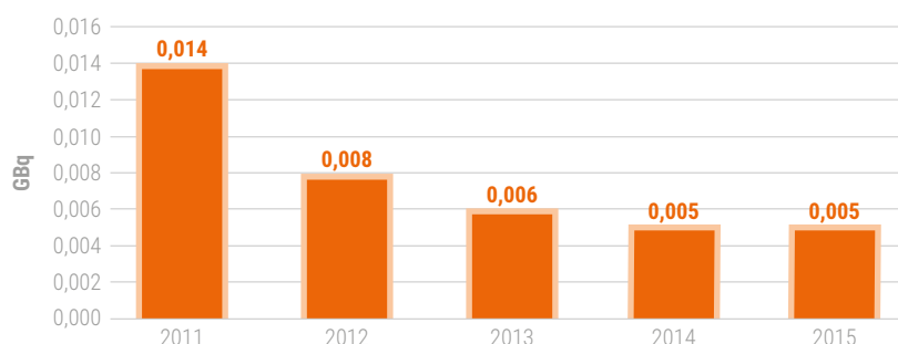
Diagramme n° 4 : Activité totale de Tritium rejetée de 2011 à 2015.
