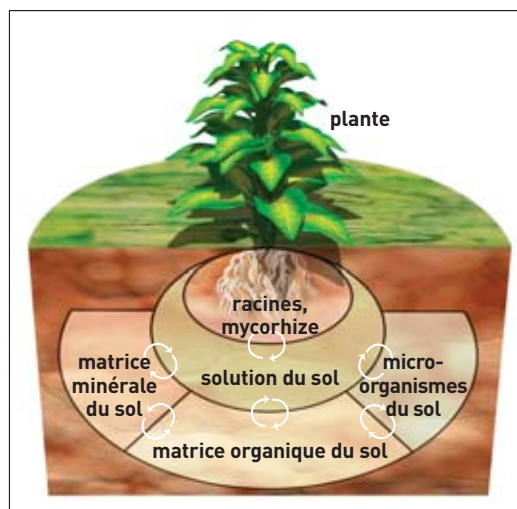
Figure. Les études de transfert des radionucléides du sol vers les plantes prennent en compte les différents compartiments du sol.
