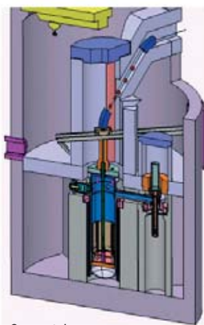
Concept de démonstrateur d'ADS de 80 MWth refroidi au gaz étudié par Framatome-ANP (Areva) dans le cadre du projet PDS-XADS.
