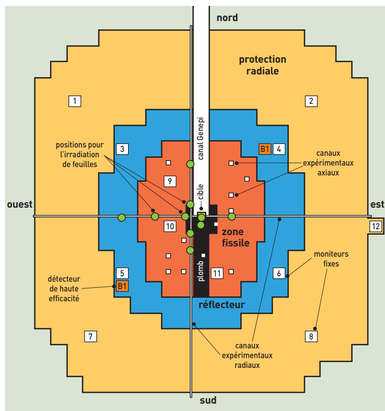
Figure 5. Coupe radiale d'un cœur MUSE-4 avec les moyens de mesure associés.
