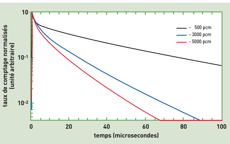
Figure 3. Réponse du cœur suite à une injection de neutrons.
