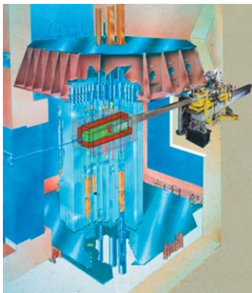
L'expérience d'ADS Muse pour l'étude de la physique des réacteurs hybrides (schéma, ci-dessus, à gauche), conduite au centre CEA de Cadarache, associe le réacteur expérimental Masurca (page de gauche) et la source de neutrons constituée par l'accélérateur Genepi (ci-dessus, à droite).
