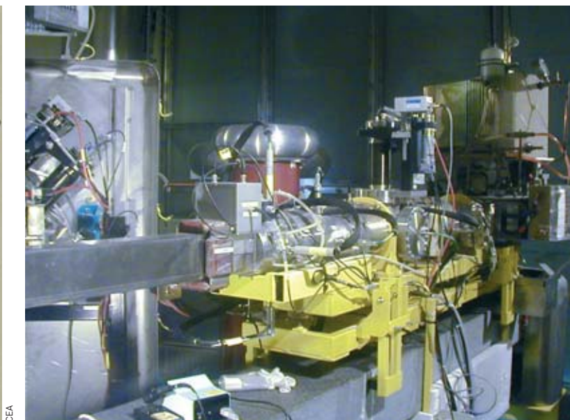
L'expérience d'ADS Muse pour l'étude de la physique des réacteurs hybrides (schéma, ci-dessus, à gauche), conduite au centre CEA de Cadarache, associe le réacteur expérimental Masurca (page de gauche) et la source de neutrons constituée par l'accélérateur Genepi (ci-dessus, à droite).
