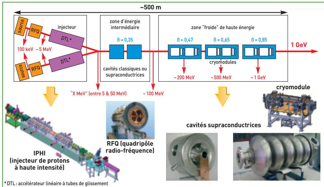
Figure 1. Les différents éléments de l'accélérateur d'un transmuteur industriel.
