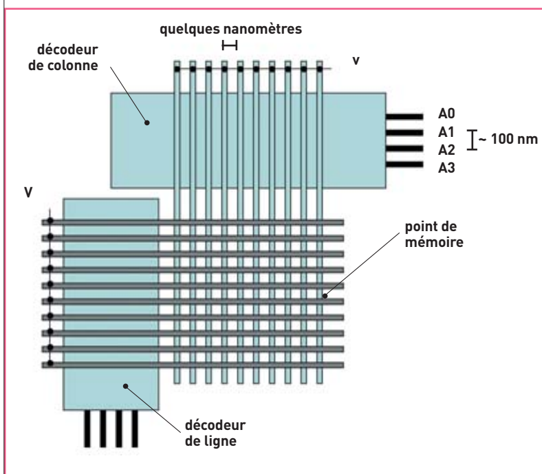
Figure 2. Schéma de principe d'une mémoire à nanofils.
