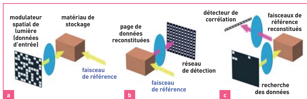
Figure 1. Les trois phases du stockage holographique de l’information.
