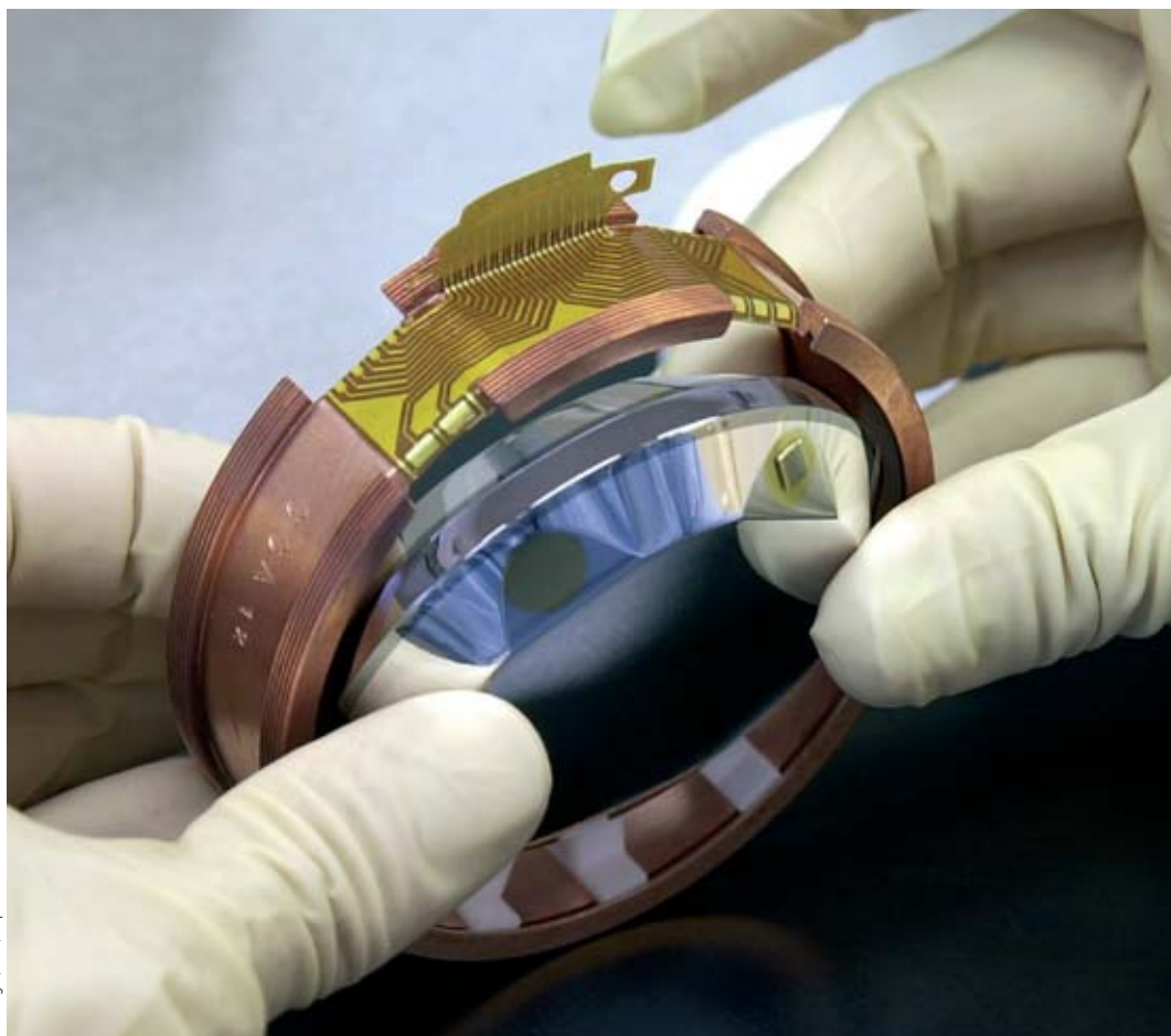
Bolomètre en germanium de 320 g et senseur thermique NTD ( Neutron Transmutation Doped ) du projet Edelweiss II.
