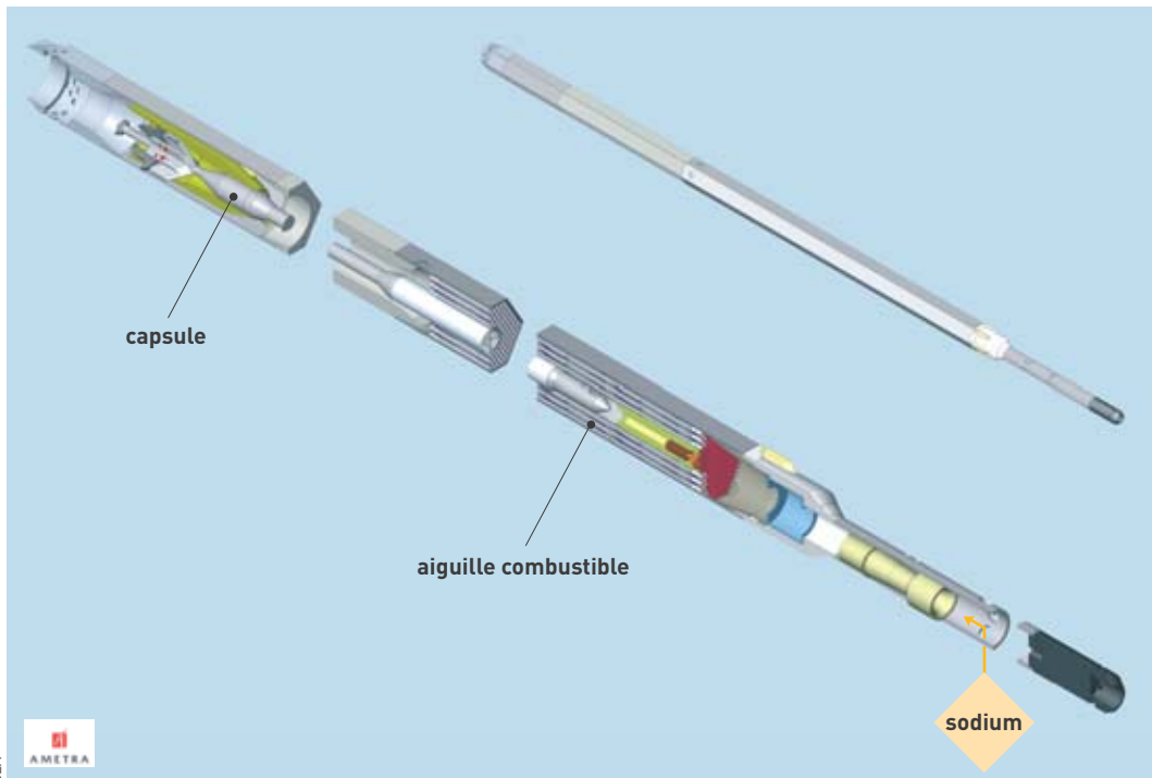
Figure 1. Dispositif d'irradiation. Les aiguilles ou les composants internes renfermant les combustibles ou les matériaux à tester sont introduits et positionnés dans la capsule expérimentale. La capsule est ensuite verrouillée dans son porteur.
