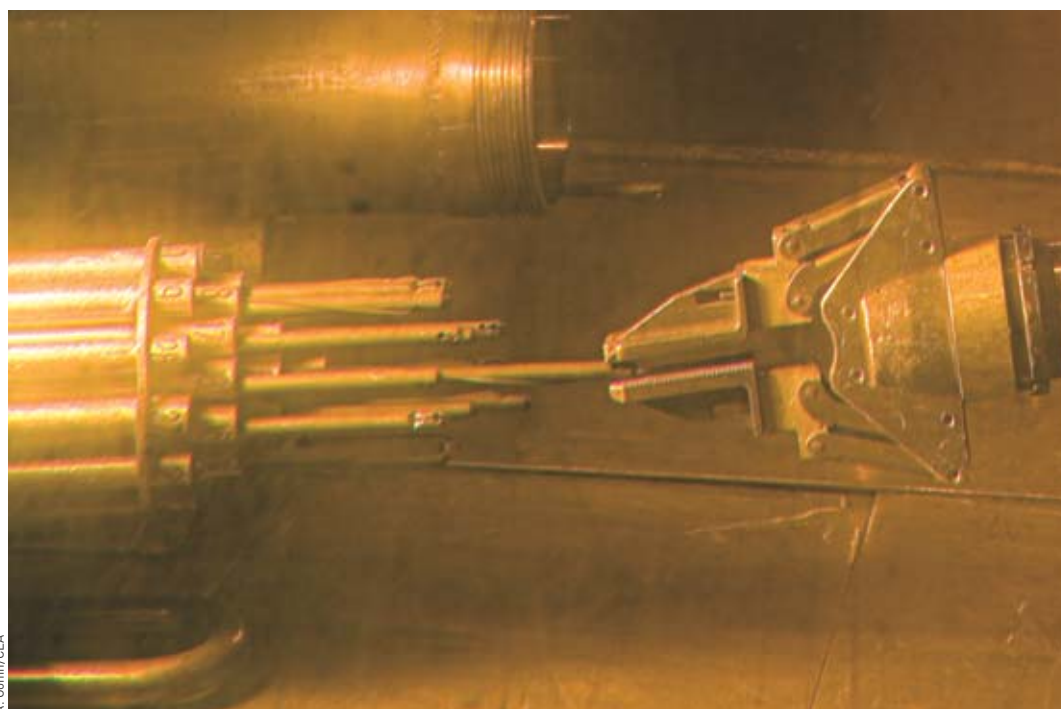
Examen non destructif d'une aiguille expérimentale Ecrix-H dans une cellule blindée de Phénix, après irradiation et refroidissement de l'expérience.
